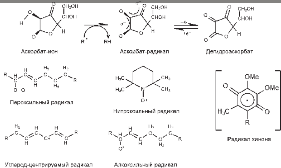
Рис. 1. Типы радикалов
